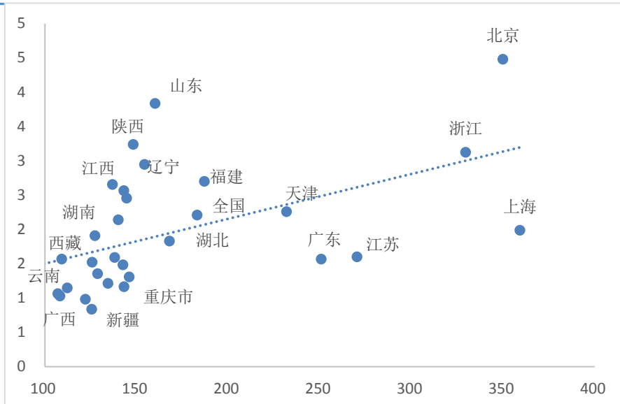
图 26：2015 年 9 月各各省支付发展指数与 2014 年人均社零总额 数据来源：2015 年中国统计年鉴（单位：万元/人）
